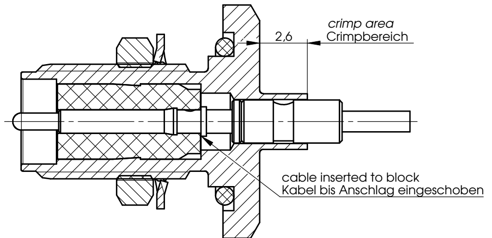
crimp insert / Crimpeinsatz: N01001A0010
